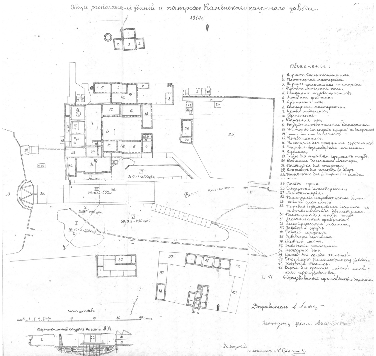
Илл. 2. План Каменского завода. 1914 г.
